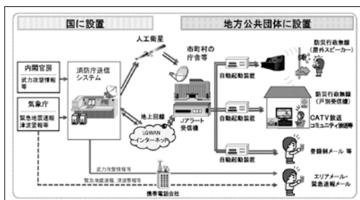
全国瞬時警報システム Jアラートの仕組み
